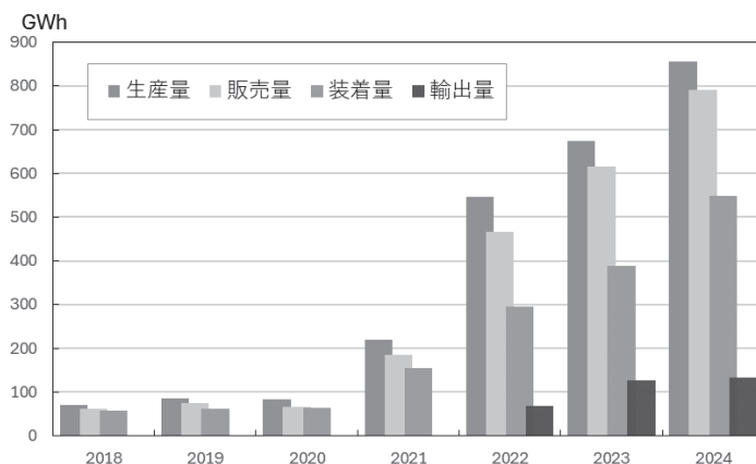
図表6 動力電池の生産、販売、実装、輸出量の推移
