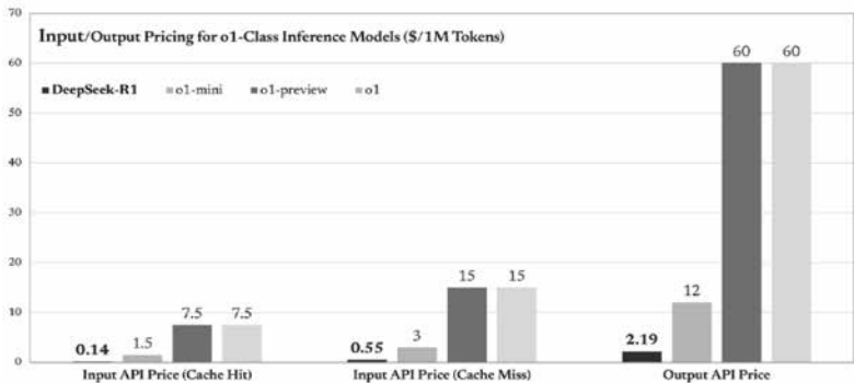
図表 3：OpenAI とのコスト比較
