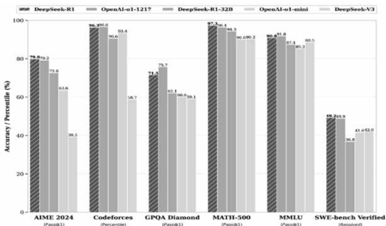
図表 2：OpenAI とのパフォーマンス比較
